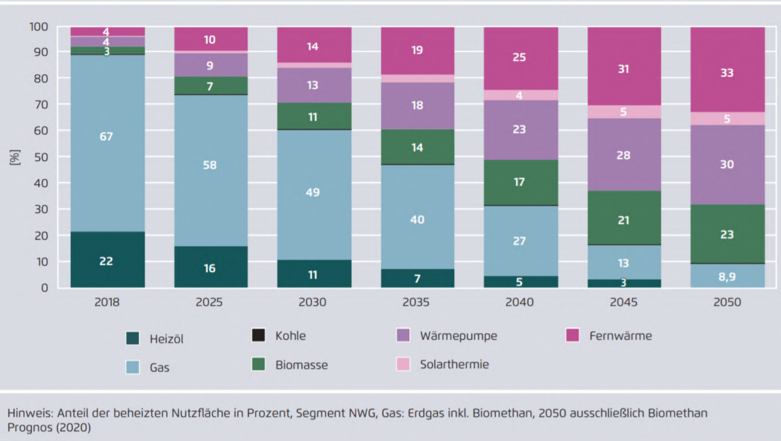
Beheizungsstruktur Gebäudefläche im GHD-Sektor
